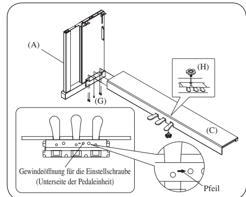
Einstellschraube (H)
